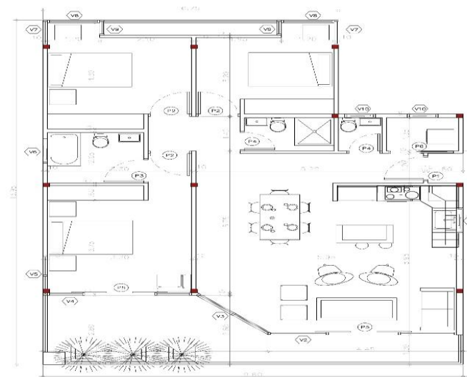
PLANTA ARQUITECTONICA TIPO A = 123 M2
