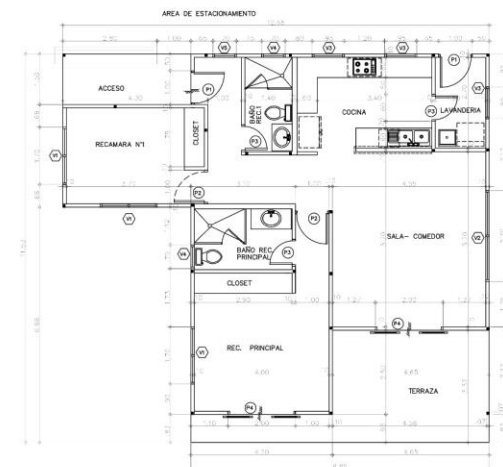
PLANTA ARQUITECTONICA MODELO VALENCIA= 130.00 M2
