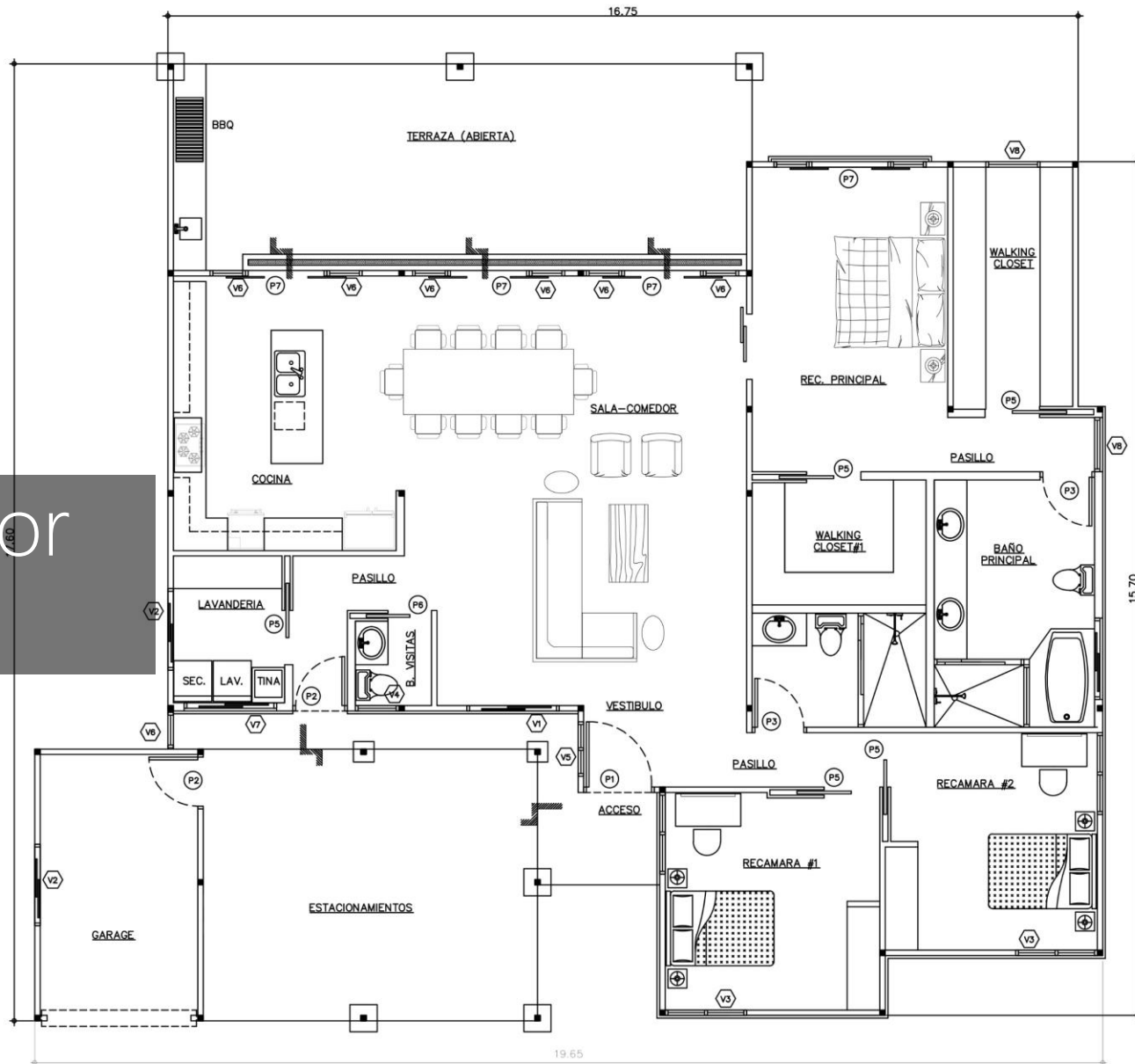
PLANTA ARQUITECTONICA CASA N°2= 290.50 M2
