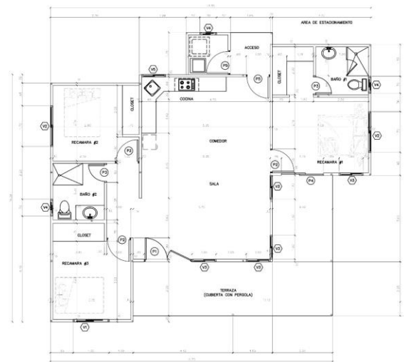
PLANTA ARQUITECTONICA MODELO SEVILLA= 150.00 M2
