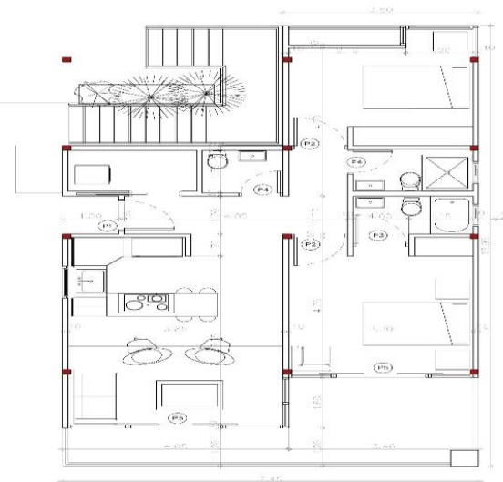
PLANTA ARQUITECTONICA TIPO B = 89 M2
