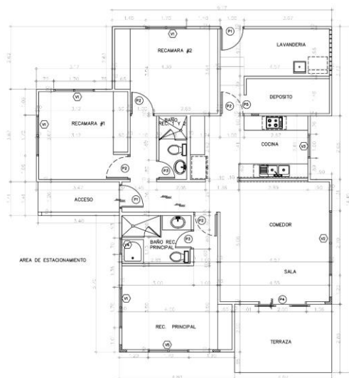
PLANTA ARQUITECTONICA MODELO MARBELLA= 150.00 M2
