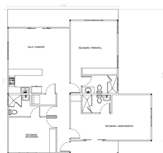
PLANTA ARQUITECTONICA MODELO CASTILLA= 160.00 M2+ESTACIONAMIENTO
