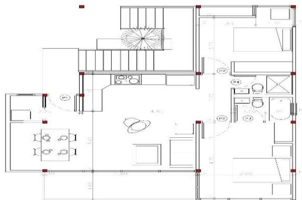
PLANTA ARQUITECTONICA TIPO C = 77 M2
